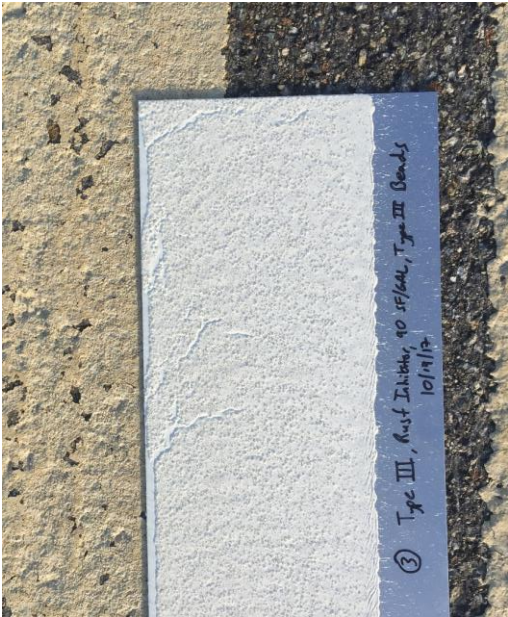
Area 3 - III RI/III
