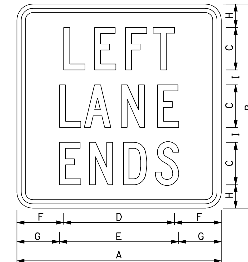
W4-2a(L)
